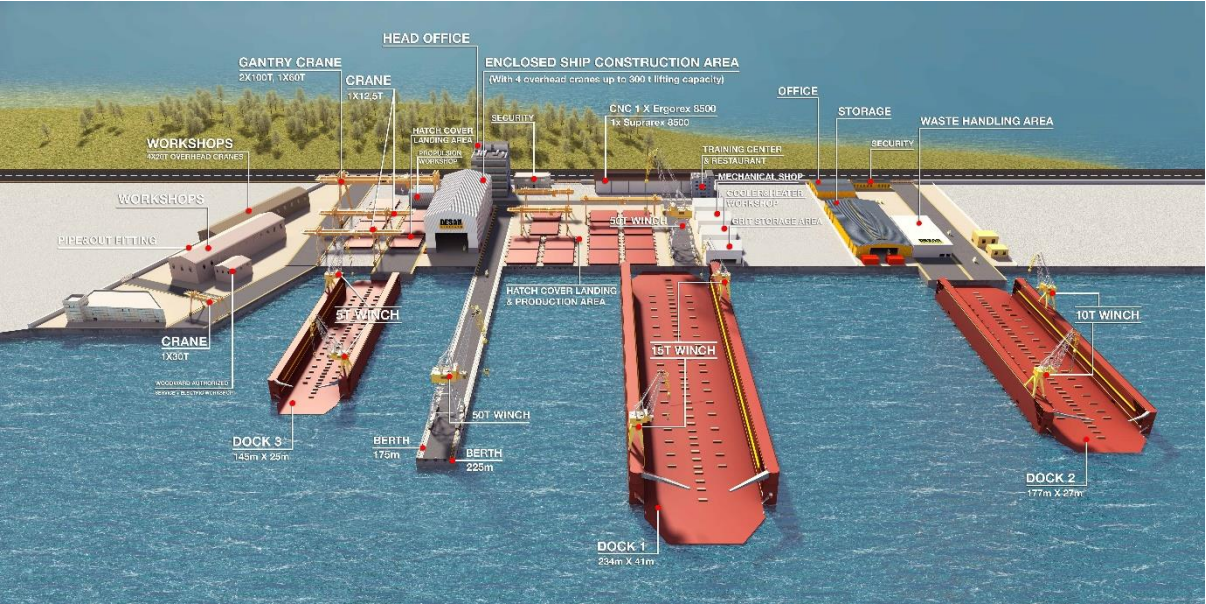
図 1 Desan Shipyard レイアウト
