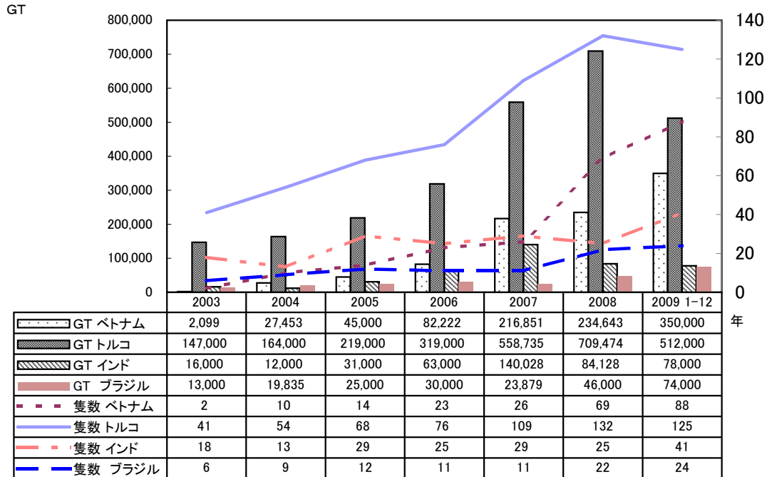
ベトナム・トルコ・インド・ブラジルの竣工量の推移
