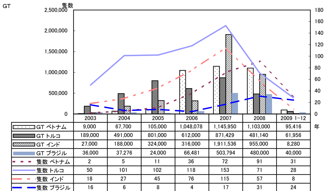
ベトナム・トルコ・インド・ブラジルの受注量の推移
